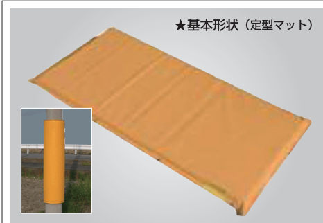
②SMS 定型タイプ size:1,800mm×900mm×t80mm 外装部：ポリエステル帆布／緩衝部：ウレタン、PE ボード 装備：ハトメ／外装形状：箱型、封筒型
