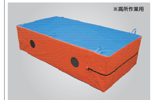
※高所作業用 ★落下対策用大型マット (SML-B2010-500-ER) size:1m×2m×0.5m／ポリエステル帆布、ウレタン、取手、他
