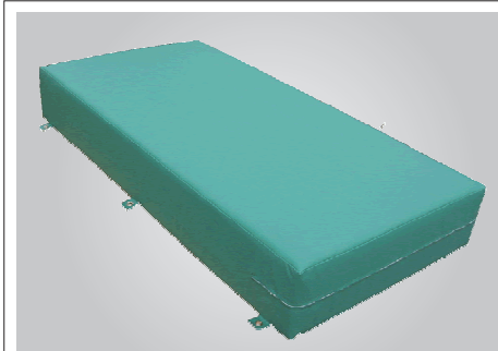
②SML 大型タイプ size:2,000mm×1,000mm×t100~300mm 外装部：ポリエステル帆布／緩衝部：ウレタン、PE ボード 装備：ハトメ／外装形状：箱型、封筒型
